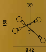
6604 N Plafoniera orientabile interamente in metallo verniciato nero con portalampada in finitura ottone invecchiato Adjustable black painted full-metal ceiling lamp with lamp holder in antique brass finish
